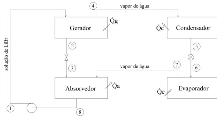
Figura 2.1. Ciclo de absorção esquemático.
