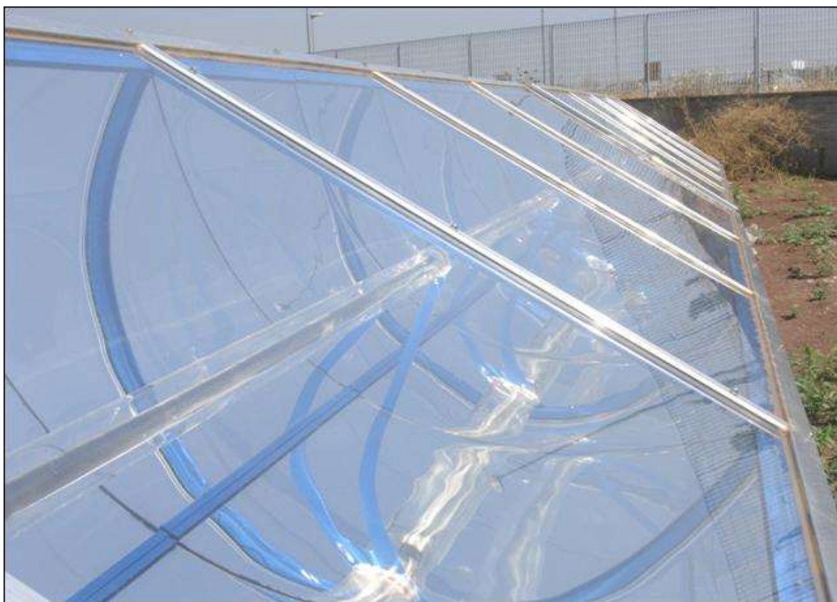
Figura 5 - Concentrador parabólico linear (Fonte: SolarPACES)
