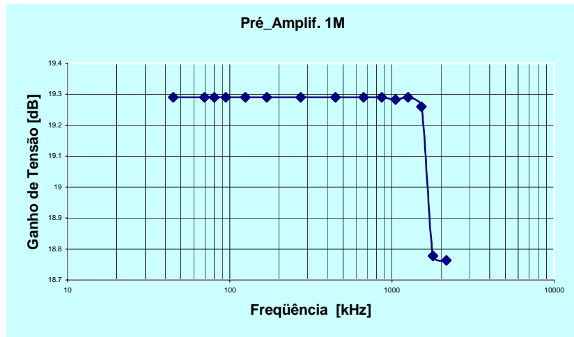
Figura 10. Resposta em frequência de pré amplificador, R_G = 1 M\Omega .
