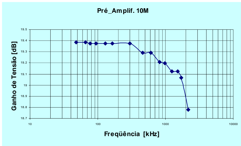
Figura 11. Resposta em frequência de pré amplificador, R_G = 10 M\Omega .
