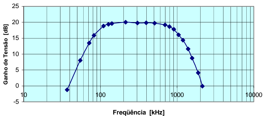
Figura 15. Curva da resposta em frequência do filtro passa banda.
