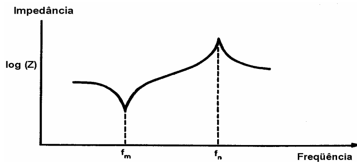
Figura 5 Característica Impedância-Frequência do cerâmico PZT ressonante.
