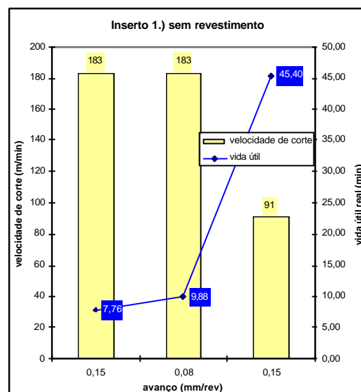
figura 13 inserto marca 1 sem revestimento
