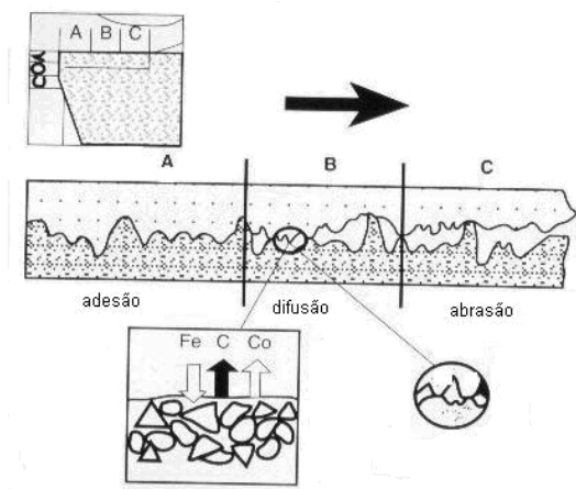
figura 1 – principais mecanismos de desgaste (adesão, abrasão, difusão)
