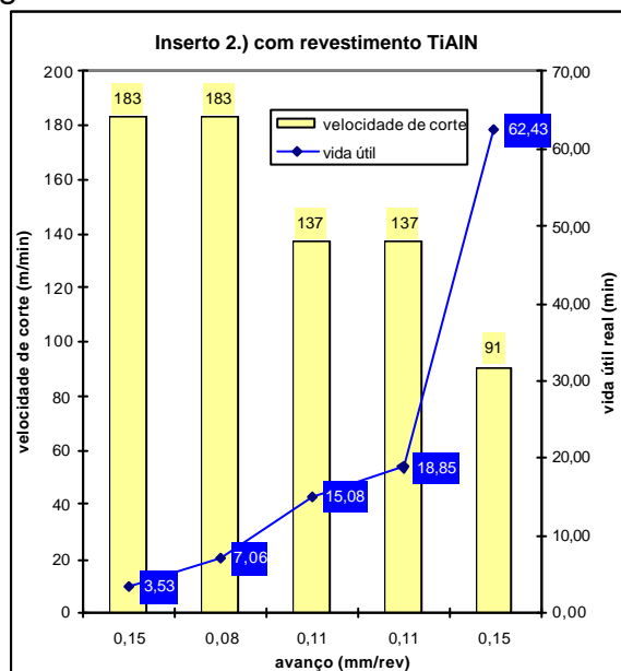
figura 14- inserto marca 2 com revestimento
