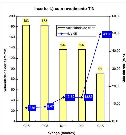
figura 12 inserto marca 1 com revestimento
