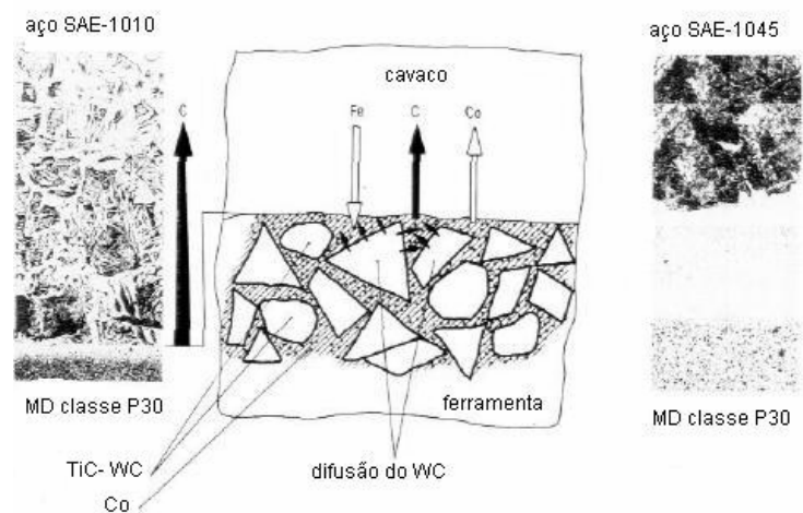
figura 2 – difusão do material da ferramenta na peça (cavaco)
