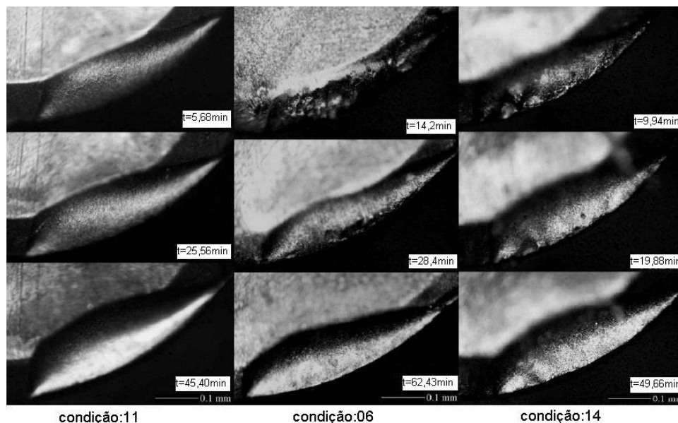
figura 5 – desenvolvimento do crateramento
