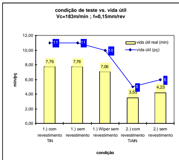
(a) – V_c=183\text{m/min} ; f=0,15\text{mm/rev}
