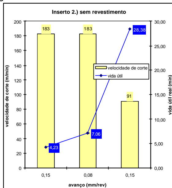
figura 15 – inserto marca 2 sem revestimento
