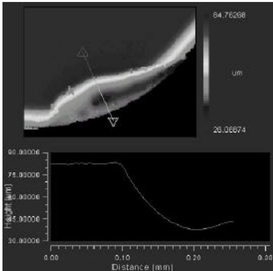
figura 6 perfil da aresta de corte condição 6
