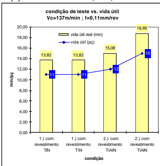
(c) - V_c=137\text{m/min} ; f=0,11\text{mm/rev}
