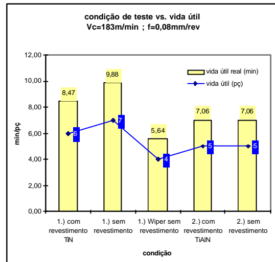
(b) – V_c=183\text{m/min} ; f=0,08\text{mm/rev}
