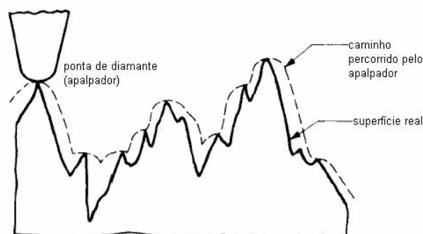
figura 4 – condição de medição (rugosidade)
